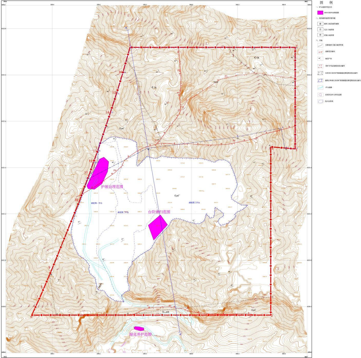
内蒙古松塔水泥有限责任公司阿左旗牛石头山水泥用石灰岩矿2025年计划治理范围图
