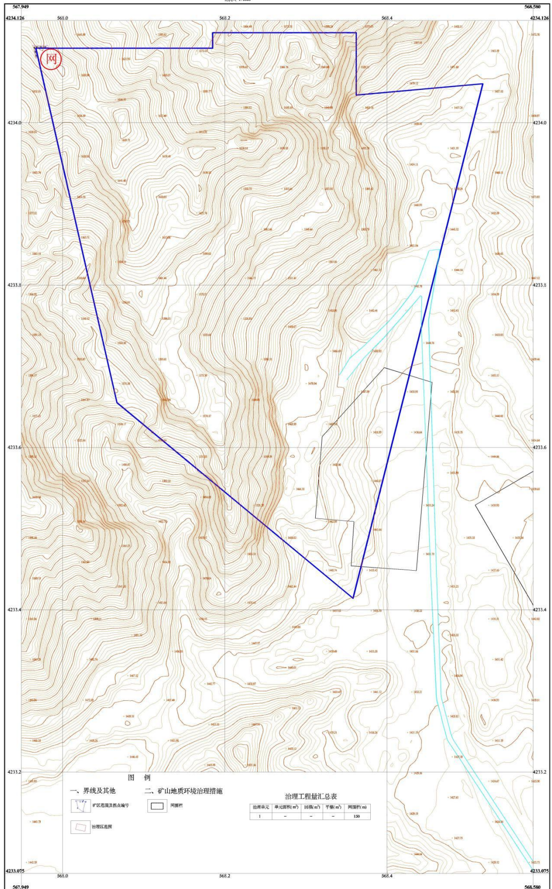
阿左旗巴润别立镇上海嘎查磨石沟建筑石料用灰岩一矿项目2025年治理计划工程部署图 比例尺 1:2000
