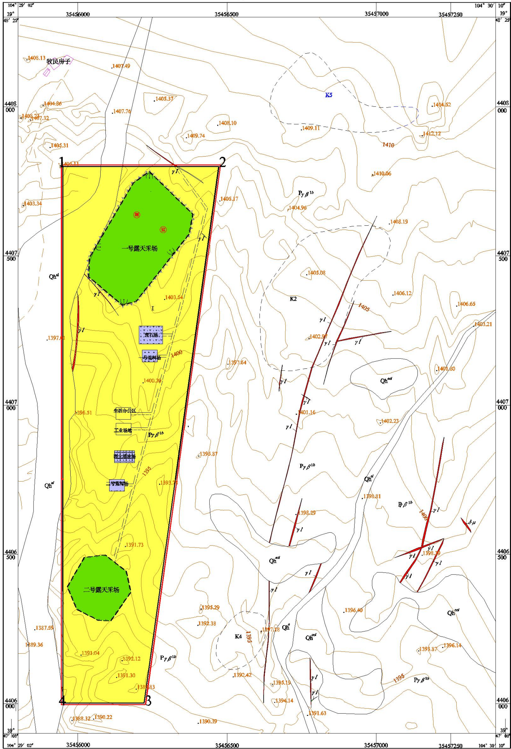
内蒙古自治区阿拉善左旗巴彦诺日公矿区昆德楚鲁一区饰面花岗岩矿矿山环境治理工程布置图
