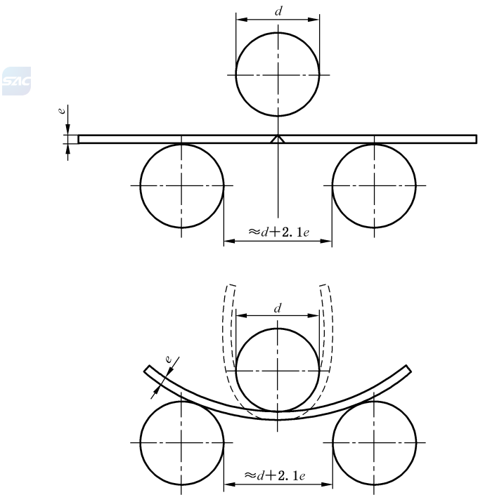
图 7 对接接头弯曲试验
